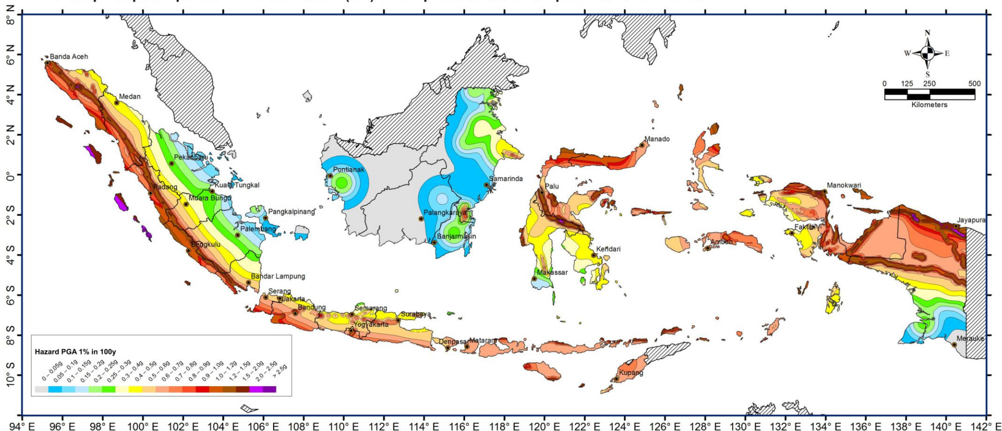
D14: Peta percepatan puncak di batuan dasar (SB) untuk probabilitas terlampaui 1% dalam 100 tahun
