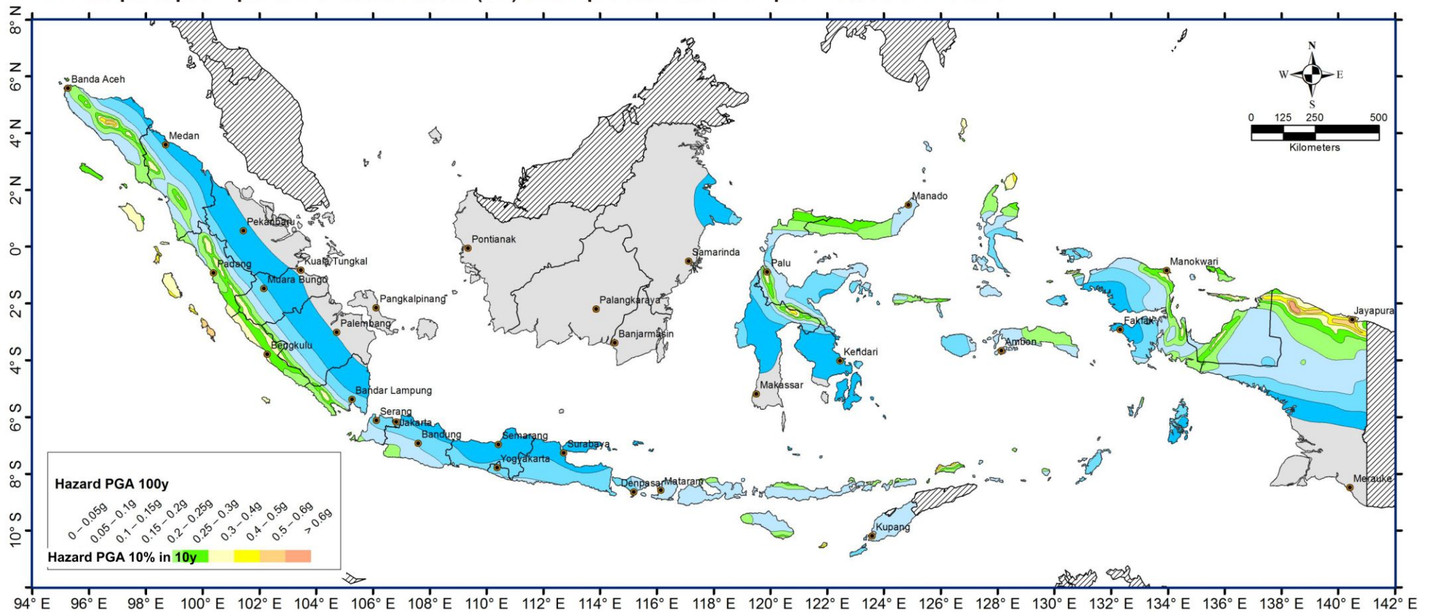
D4: Peta percepatan puncak di batuan dasar (SB) untuk probabilitas terlampaui 10% dalam 10 tahun
