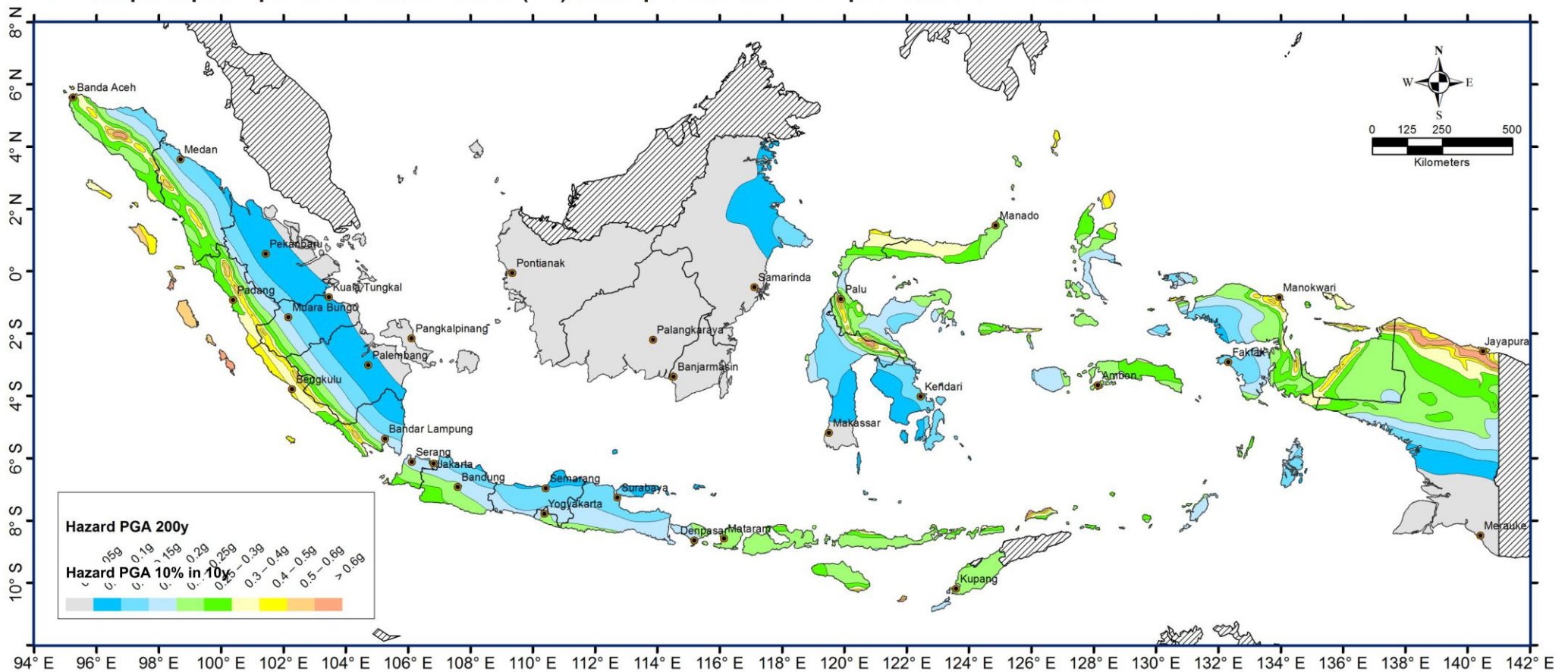
D5: Peta percepatan puncak di batuan dasar (SB) untuk probabilitas terlampaui 5% dalam 10 tahun
