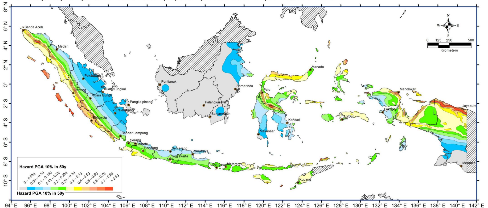
D6: Peta percepatan puncak di batuan dasar (SB) untuk probabilitas terlampaui 10% dalam 50 tahun
