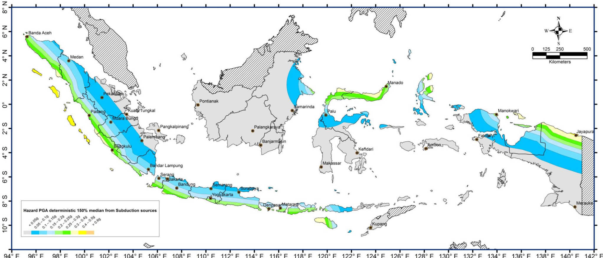
D2: Peta percepatan puncak di batuan dasar (SB) deterministik akibat sumber gempa Subduksi dengan 84-percentile (150% Median)
