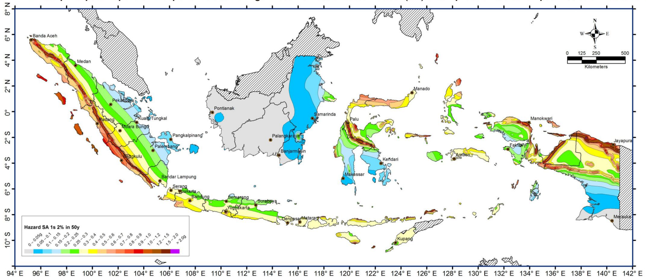
D12: Peta percepatan spektrum respons 1.0 detik dengan redaman 5% di batuan dasar (SB) untuk probabilitas terlampaui 2% dalam 50 tahun
