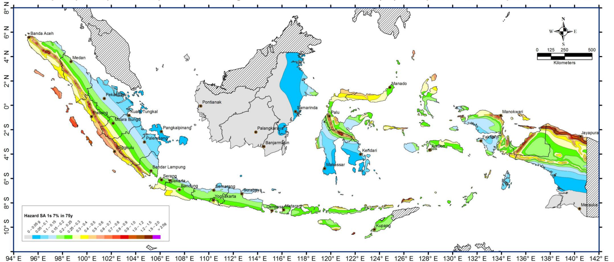
D9: Peta percepatan spektrum respons 1.0 detik dengan redaman 5% di batuan dasar (SB) untuk probabilitas terlampaui 7% dalam 75 tahun
