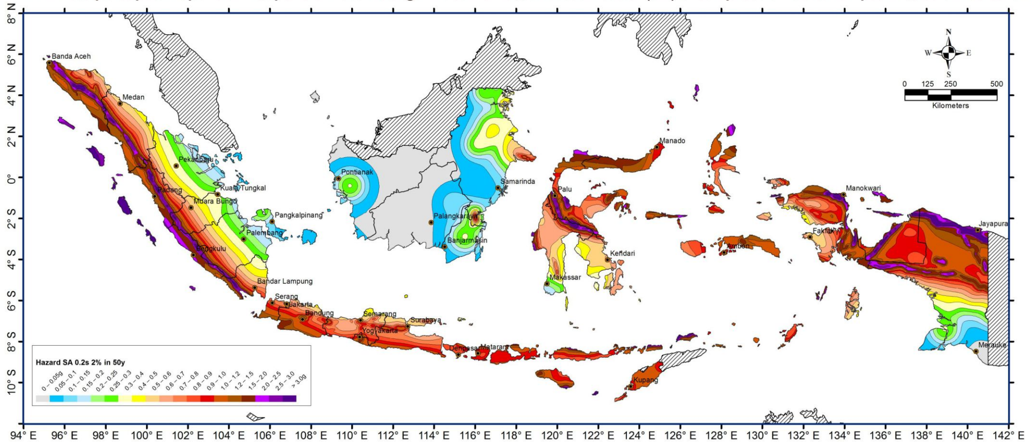
D11: Peta percepatan spektrum respons 0.2 detik dengan redaman 5% di batuan dasar (SB) untuk probabilitas terlampaui 2% dalam 50 tahun
