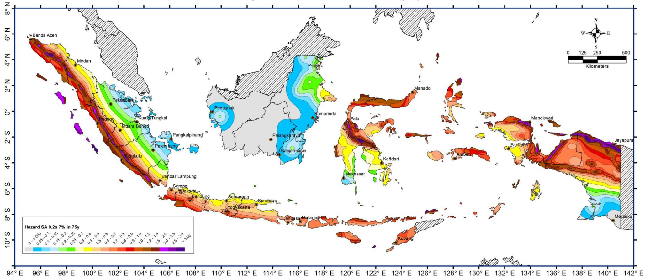
D8: Peta percepatan spektrum respons 0.2 detik dengan redaman 5% di batuan dasar (SB) untuk probabilitas terlampaui 7% dalam 75 tahun
