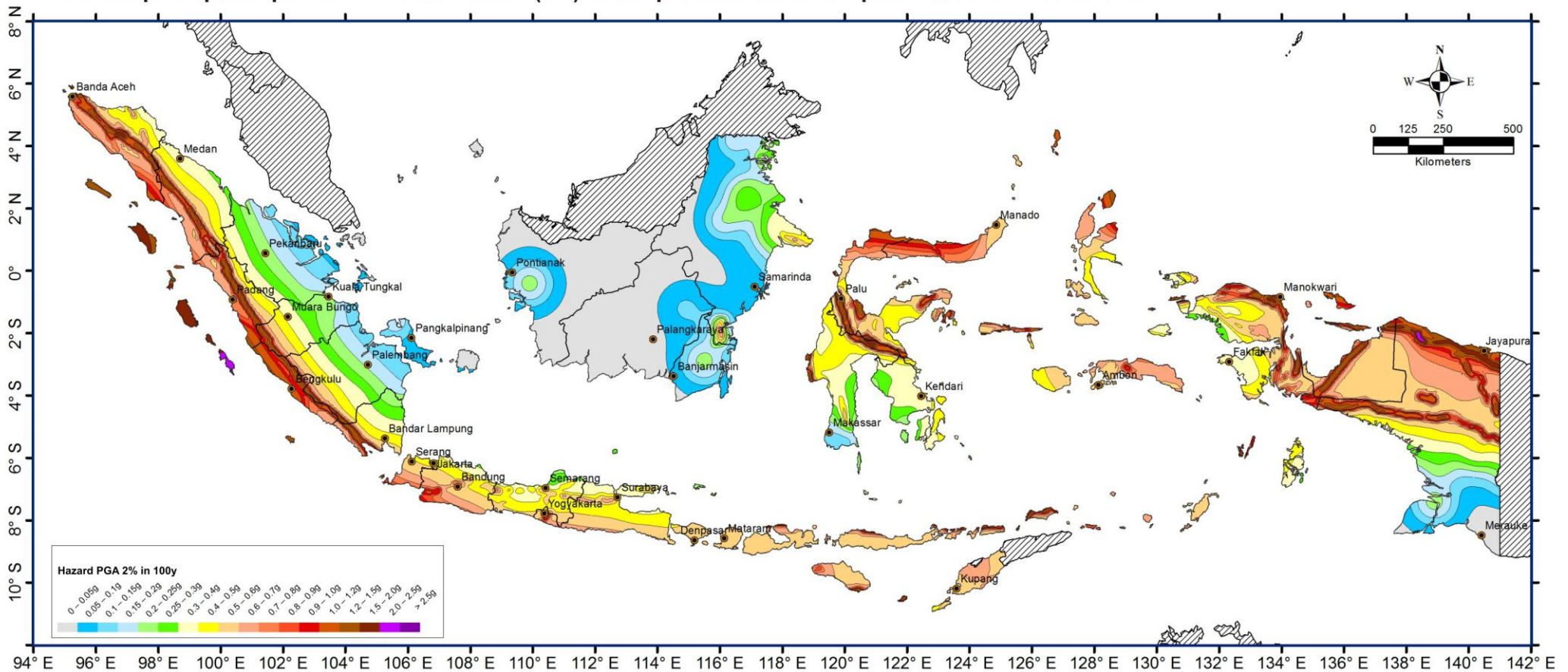
D13: Peta percepatan puncak di batuan dasar (SB) untuk probabilitas terlampaui 2% dalam 100 tahun
