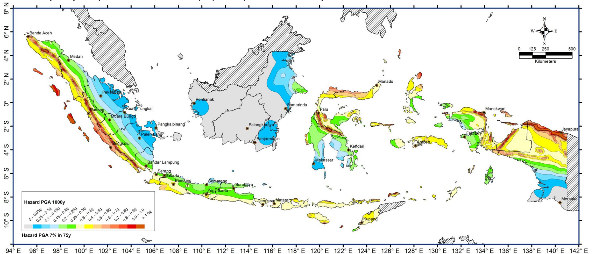
D7: Peta percepatan puncak di batuan dasar (SB) untuk probabilitas terlampaui 7% dalam 75 tahun
