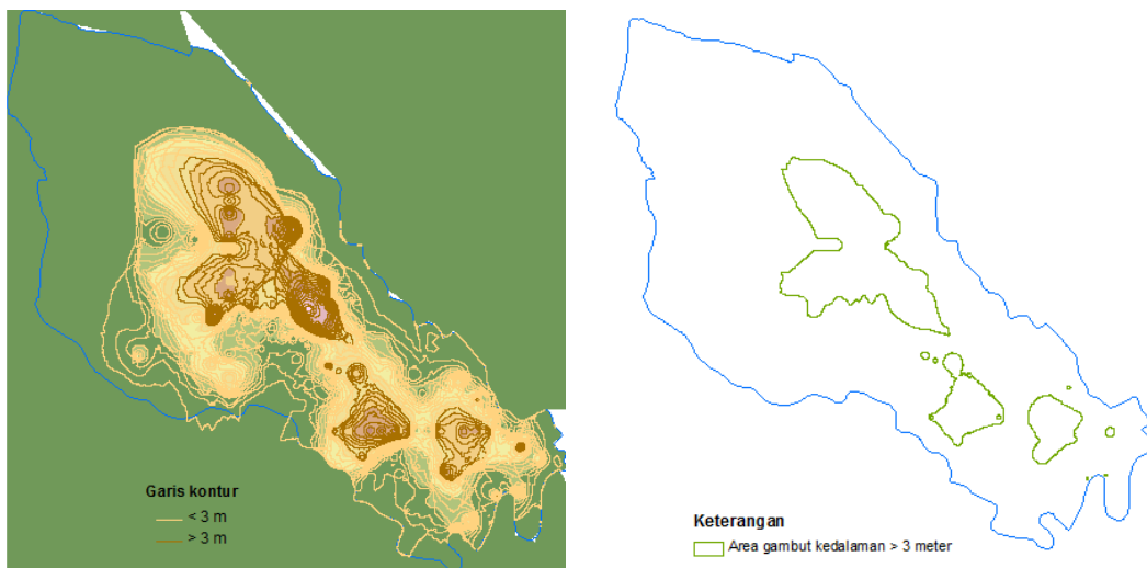
Gambar 5. Hasil identifikasi dan delineasi kontur dengan kedalaman 3 m
