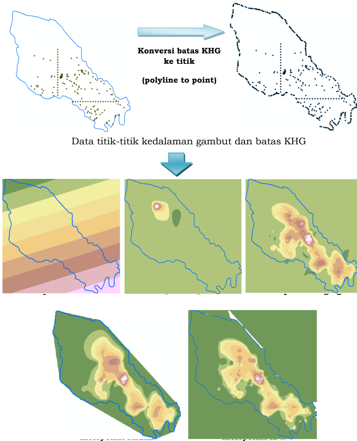
Gambar 3. Hasil kegiatan interpolasi berbagai Metode Interpolasi
