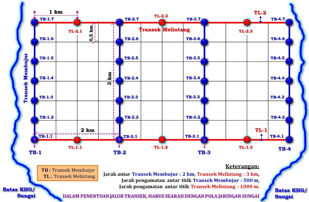
Gambar 1. Penyebaran titik sampel secara sistematis (metode sistem Grid)
