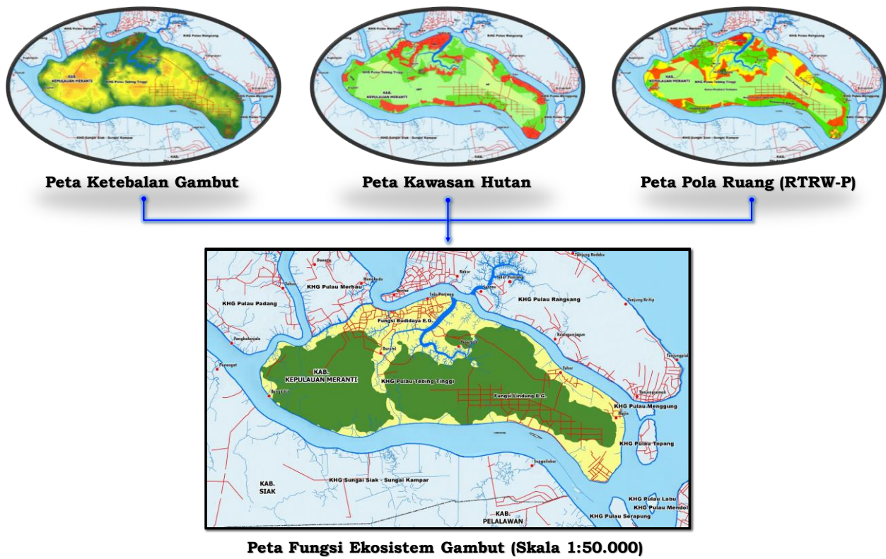
Gambar 1. Tahapan Dalam Proses Integrasi Data Penetapan Fungsi Ekosistem Gambut (Fungsi Lindung dan Fungsi Budidaya) Skala 1:50.000
