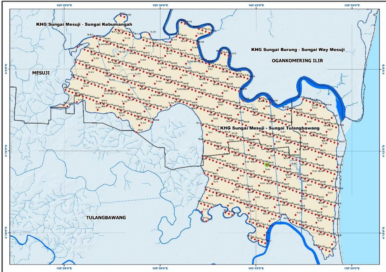
Gambar 51. Contoh Peta Transek dan Titik Pengamatan Inventarisasi Karakteristik Ekosistem Gambut (skala 1:50.000)
