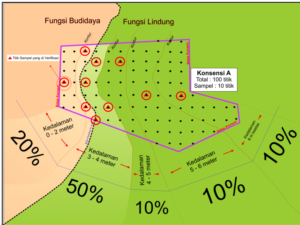
Gambar 2. Verifikasi lapangan pada areal konsesi/perizinan dengan fungsi lindung ekosistem gambut yang lebih luas dari fungsi budidaya ekosistem gambut
