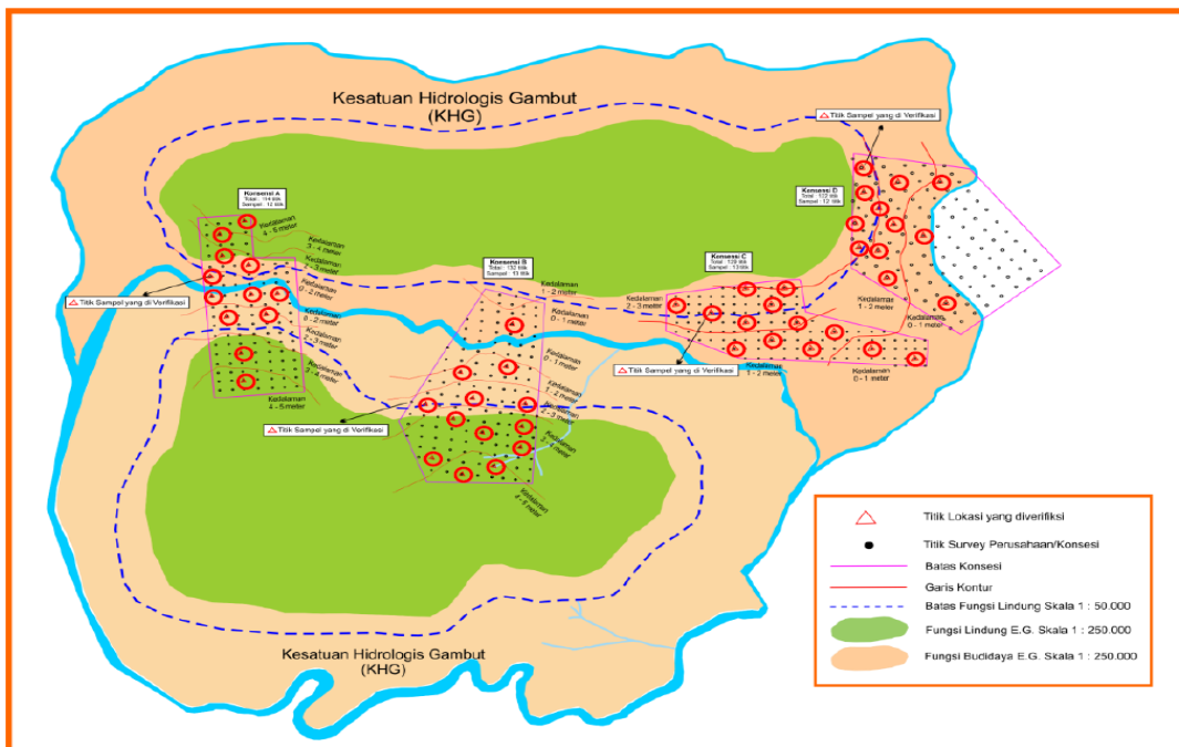
Gambar 6. Verifikasi lapangan pada beberapa areal konsesi/perizinan yang memotong fungsi lindung dan fungsi budidaya ekosistem gambut dalam 2 (dua) kesatuan hidrologis gambut atau lebih
