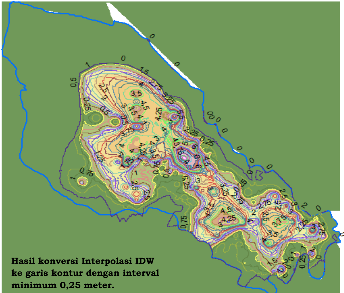
Gambar 4. Kenampakan garis kontur kedalaman gambut dari hasil interpolasi data titik pengamatan lapangan kedalaman gambut
